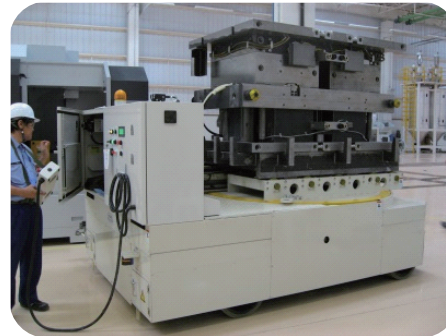
軌条・床上兼用運搬台車 最大積載重量 15t
